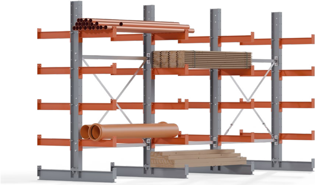
Kragarme beidseitig
